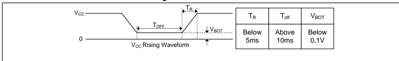
Figure 5.1 POR Condition
